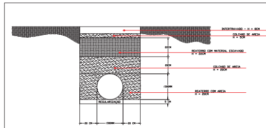
ENCANAMENTO DRENAGEM - DETALHAMENTO
